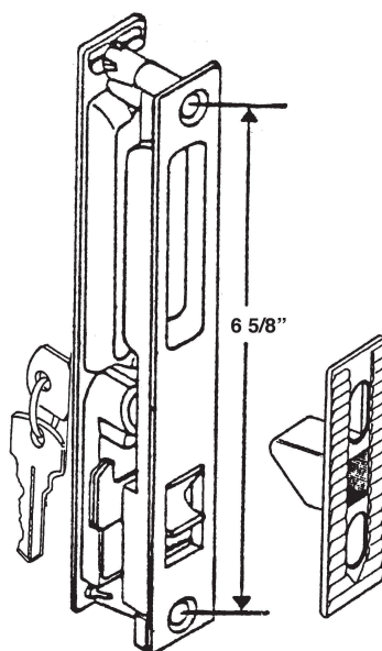
#8061 PATIO DOOR LOCK K CAM
