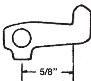
#8061 PATIO DOOR LOCK K CAM
