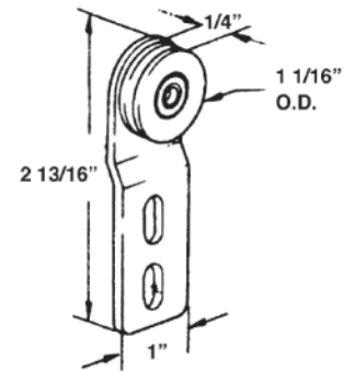
#669 PREMIER SCREEN DOOR ROLLER ASSY
