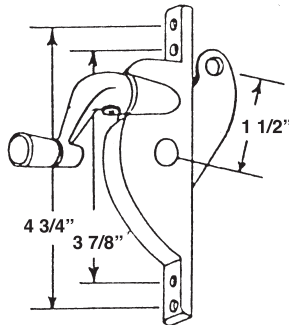
#789 D-7 L.H. JTW OPERATOR
