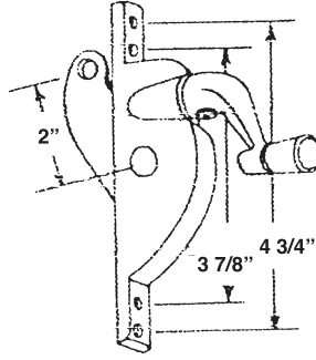
#790 D-8 R.H. JTW OPERATOR
