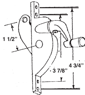
#788 D-7 R.H. JTW OPERATOR
