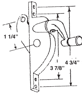
#786 LUDMAN OPERATOR R.H.
