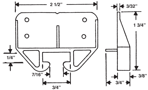
#416 DOOR TRACK SLIDE GUIDE
