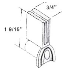
#495 SCREEN DOOR GUIDE
